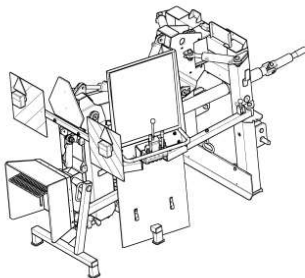
FZ 560T-M
